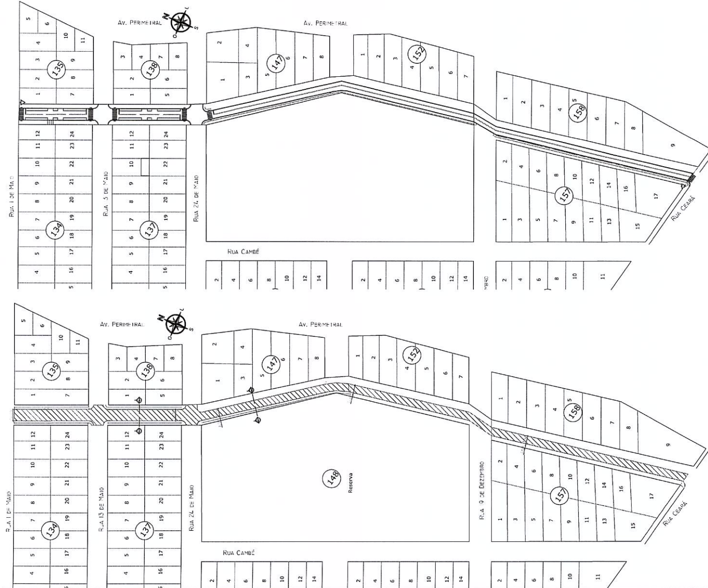
PLANTA BAIXA PAVIMENTAÇÃO E SINALIZAÇÃO HORIZONTAL E VERTICAL ESCALA 1:1200
